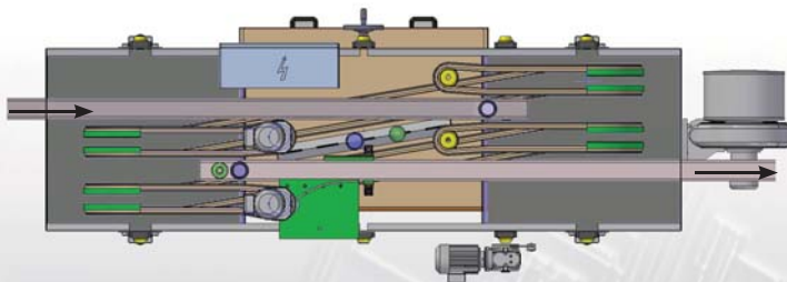
Durch die gerade Übergabe auf angestellte Transportsysteme wird ein Umfallen der Gebinde vermieden.
